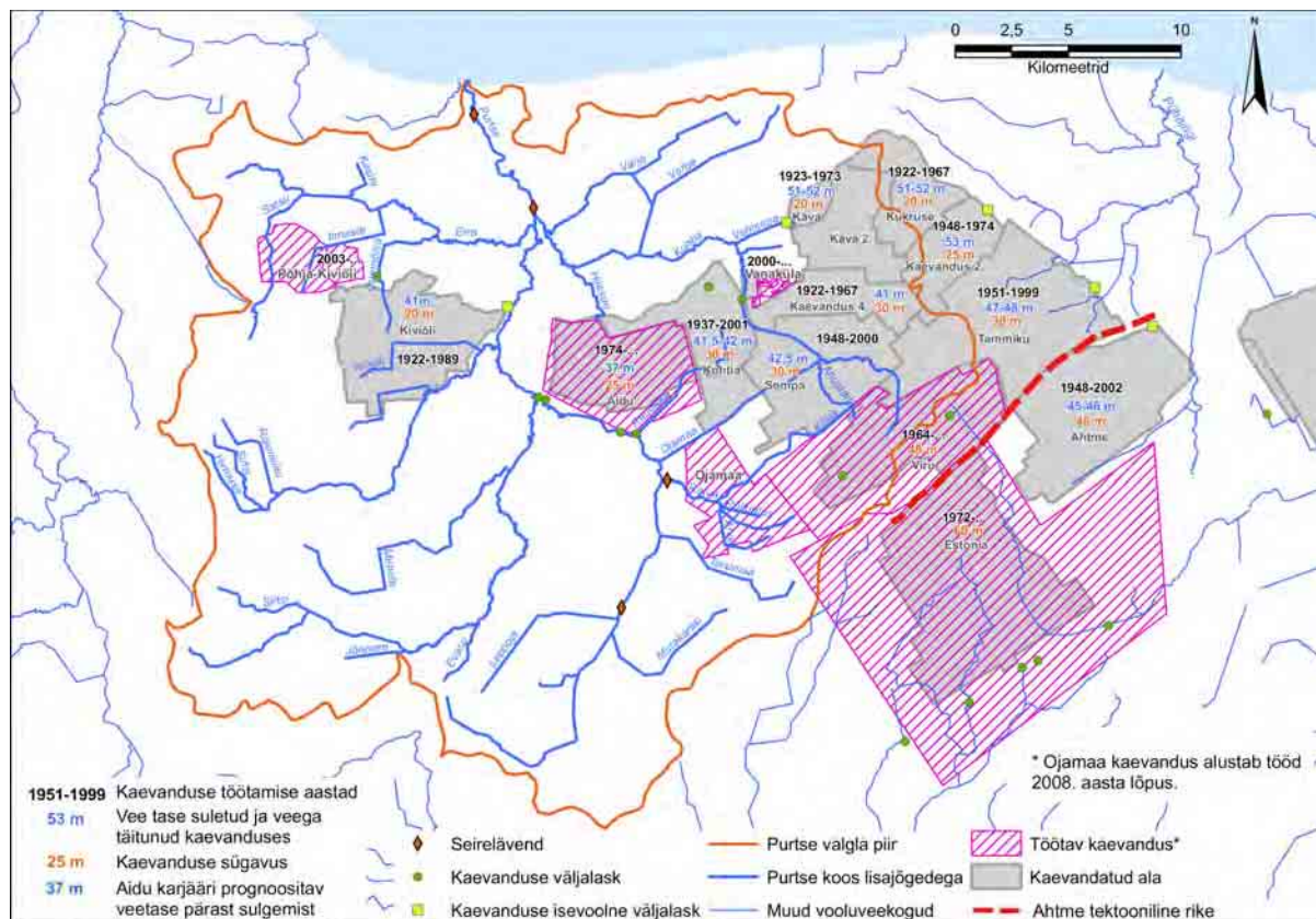
Joonis 2 Põlevikivi kaevandamine ning Purtse valgla (veetasemed on 2004 seisuga)
