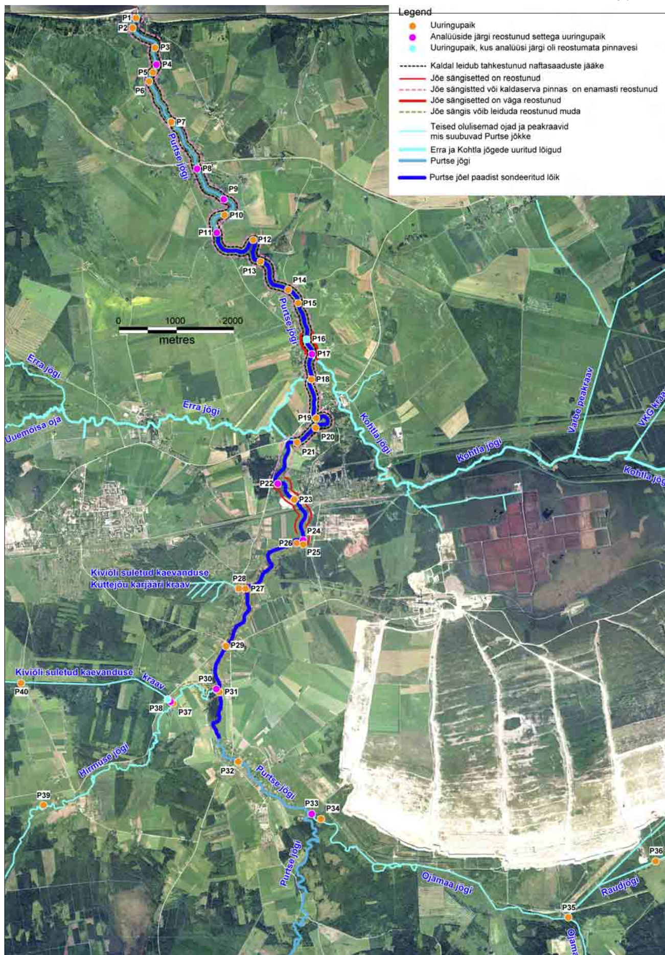
Joonis 7 Purtse jõe uuringupunktide paiknemine
