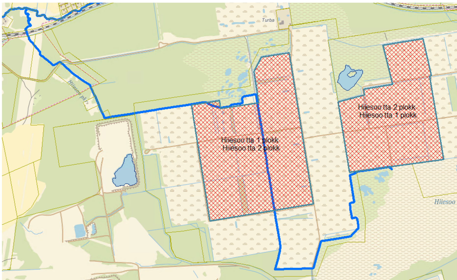
Joonis 1. Hiiesoo peakraavi (keskkonnaregistri kood VEE1071300) asukoht ümberhinnatavate plokkide piirkonnas.
