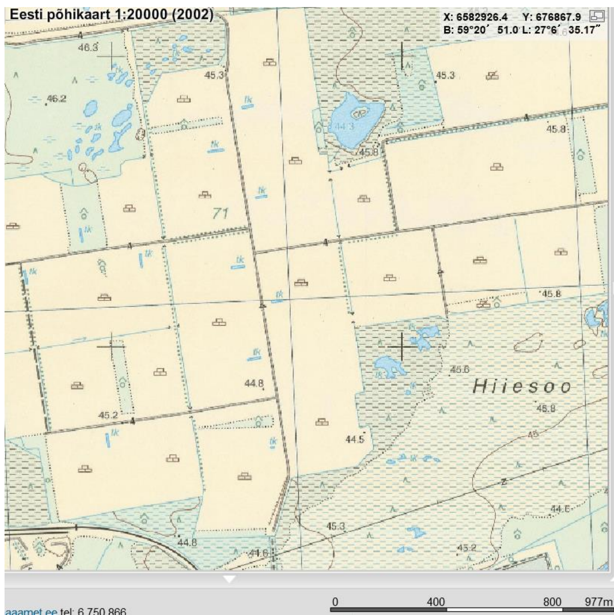
Joonis 4. Hiiesoo mäeeraldise ala 2002. a Eesti põhikaardil (Maa-amet). Turbatootmisala idasuunalise laienemise käigus on rajatud ka Hiiesoo peakraavi idapoolsem lõik.
