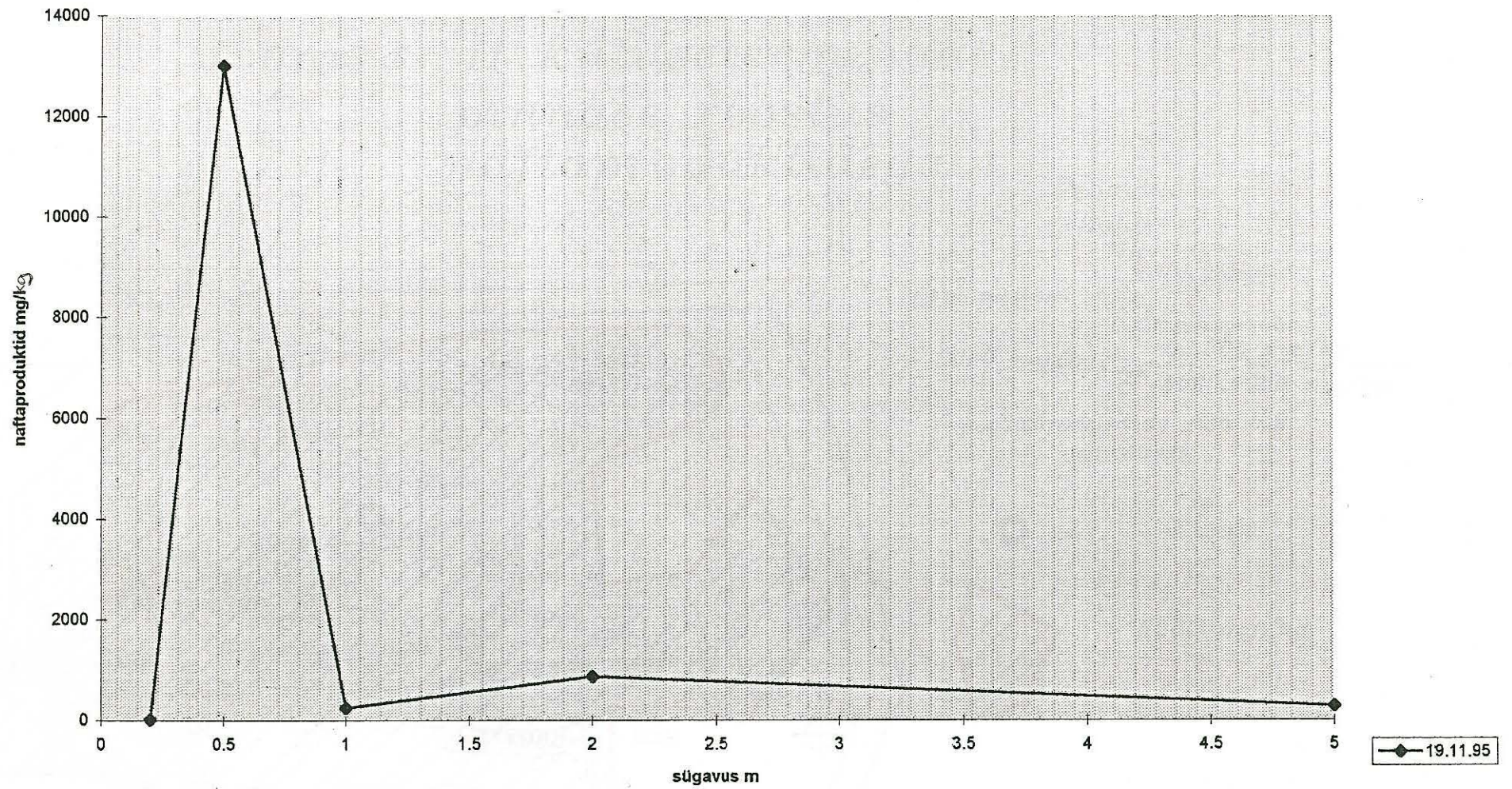
Joonis 7 PA 7 naftaproduktid pinnases, II kütuseterminaal
